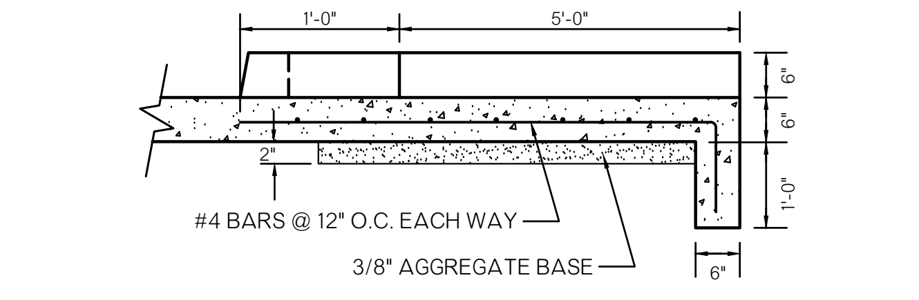
SECTION A-A
